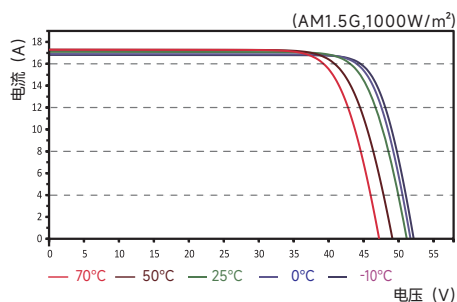
不同电池温度下, I-V曲线图
