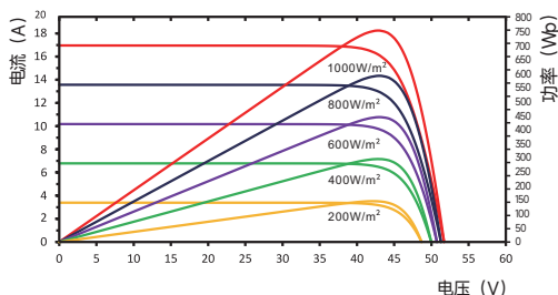
不同辐照度下, I-V曲线图
